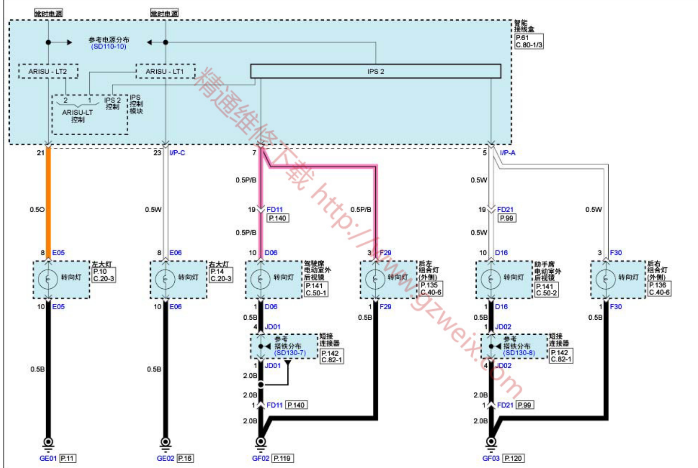
转向灯 &amp; 危险警告灯(3)
